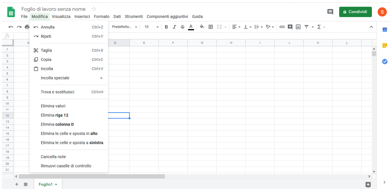
Figura 1: Menu Modifica
