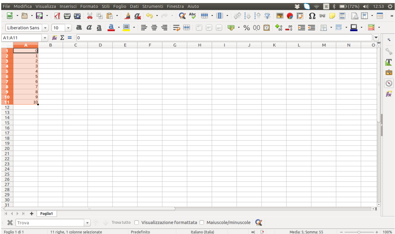
Figura 1: Riempimento automatico
