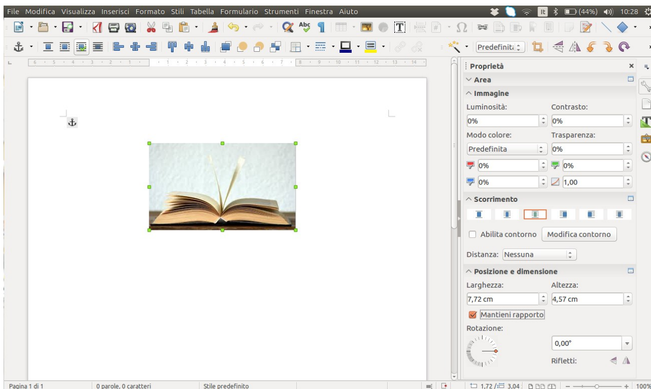
Figura 1: Ridimensionare un'immagine
